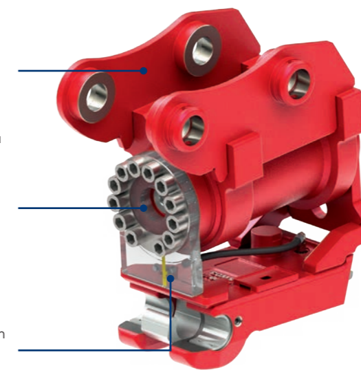
Tilt-Schnellwechsler mit baggerseitiger Direktaufhängung
